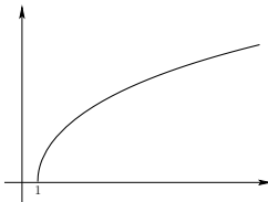
Argumento do cosseno hiperbólico
