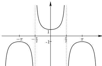
Secante
