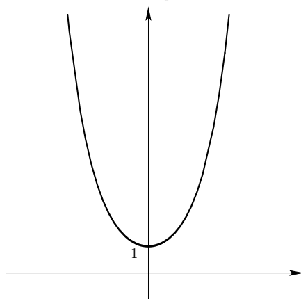
Cosseno hiperbólico
