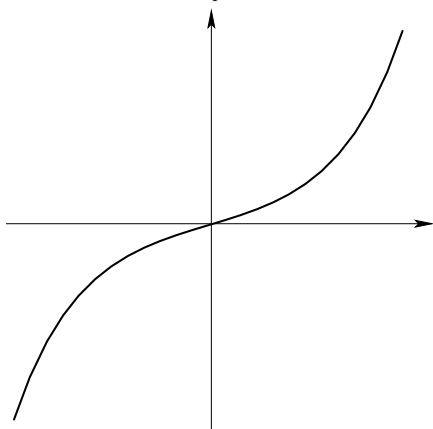
Seno hiperbólico
