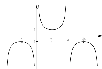
Cossecante
